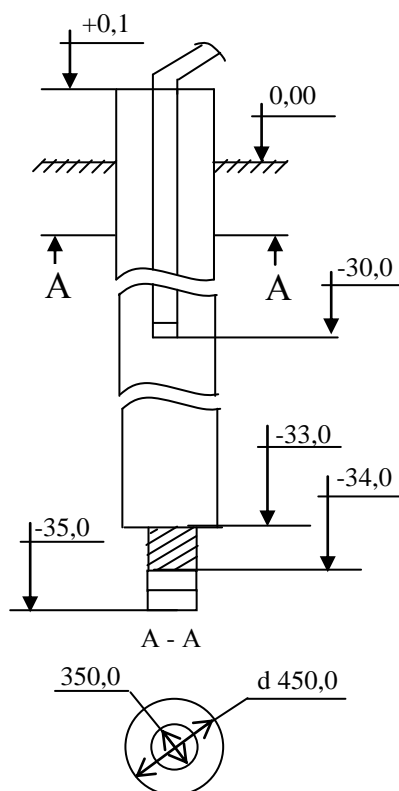
Рисунок 2 – Принципиальная схема установки водоподъемного оборудования в скважине сельского населенного пункта села Золотое
