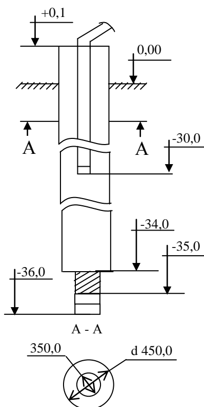
Рисунок 3 – Принципиальная схема установки водоподъемного оборудования в д. Десятый Октябрь
