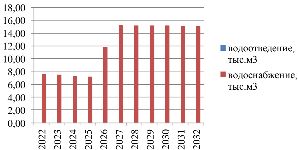
Рисунок 18 – Перспективный баланс централизованного водоснабжения и водоотведения сельского населенного пункта села Садовод
