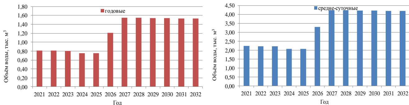
Рисунок 14 – Сведения о годовых и среднесуточных фактических и планируемых потерях питьевой воды при ее транспортировке
