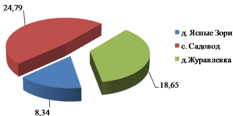
Рисунок 5 - Территориальный баланс питьевой воды по технологическим зонам за 2021 г.
