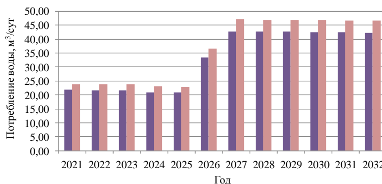
Рисунок 11 – Фактическое и ожидаемое среднесуточное и максимальное потребление питьевой воды
