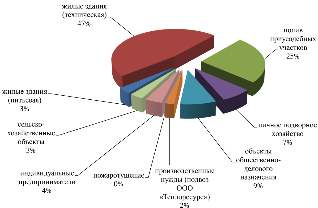
Рисунок 6 – Развернутый годовой структурный баланс реализации воды
